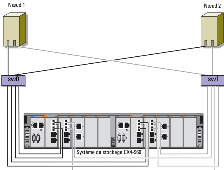
Figure 2-2. Câblage d'un cluster Fibre Channel Dell/EMC connecté à un SAN
