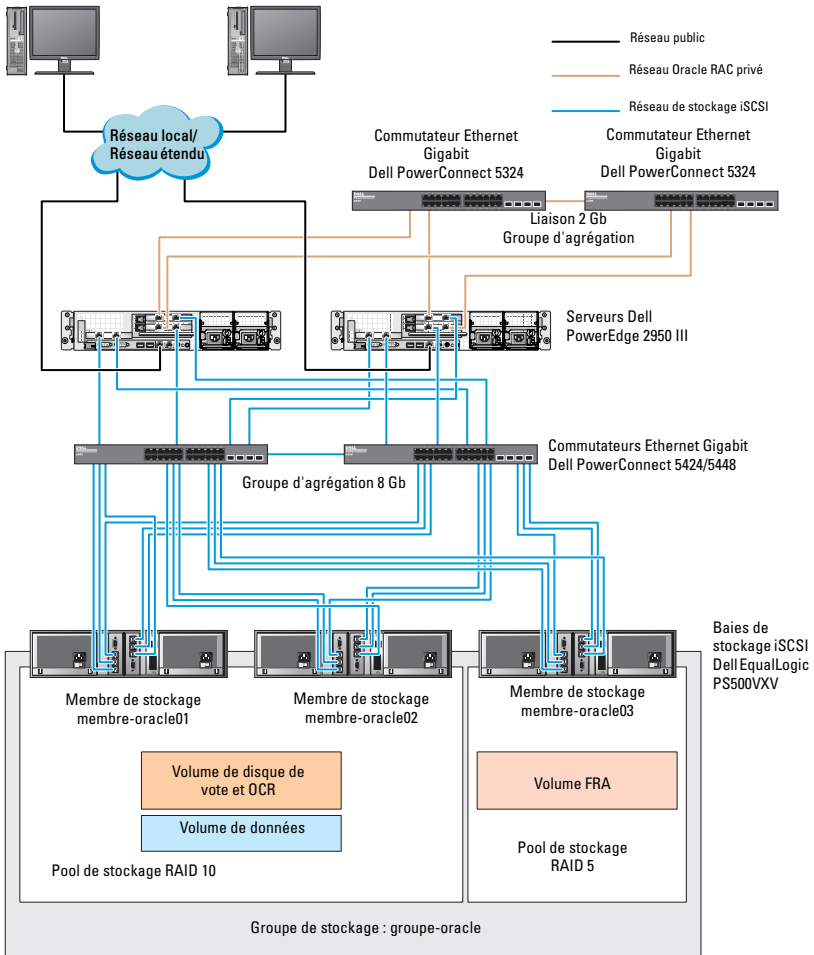
Figure 5-2. Exemple de configuration d'un cluster Oracle RAC avec trois baies PS500XV
